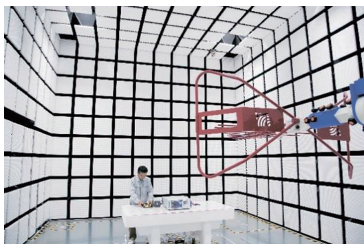
EMC 試験室（電波暗室）
